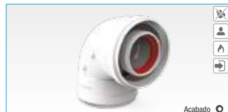
Codo coaxial 90° Hembra - Hembra Ø80 / Ø110 (Aluminio lacado)
